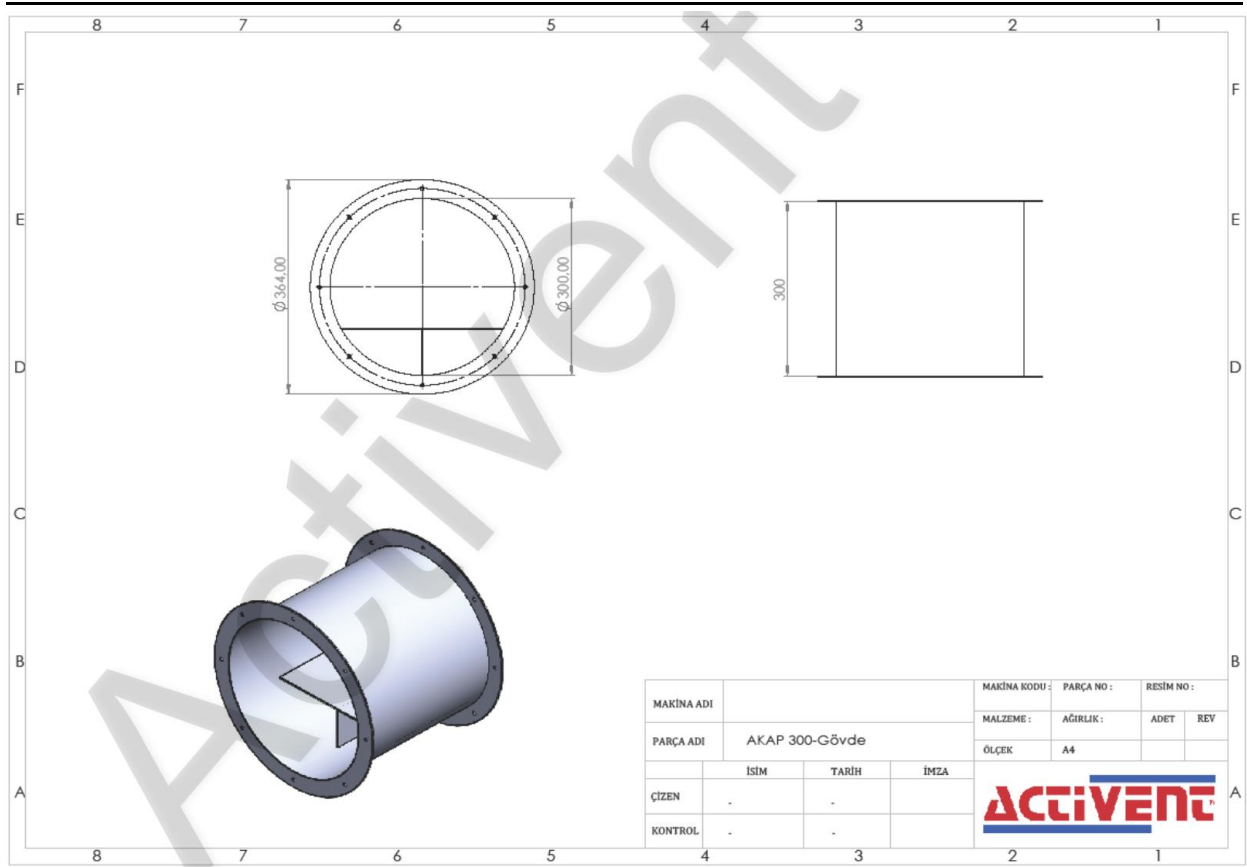
Şekil 2: Fan karkası detayları
