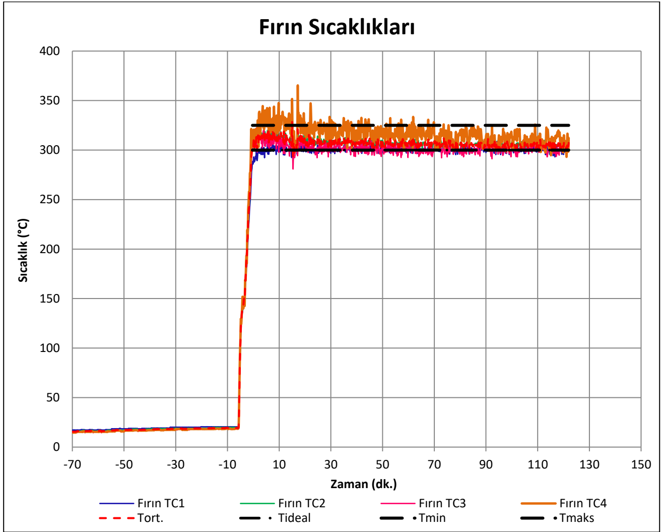
Şekil A1: Fırın sıcaklıkları
