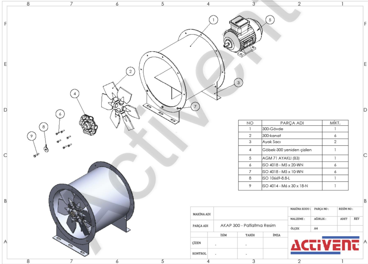
Şekil 1: Test numunesinin patlatılmış görünüşü.
