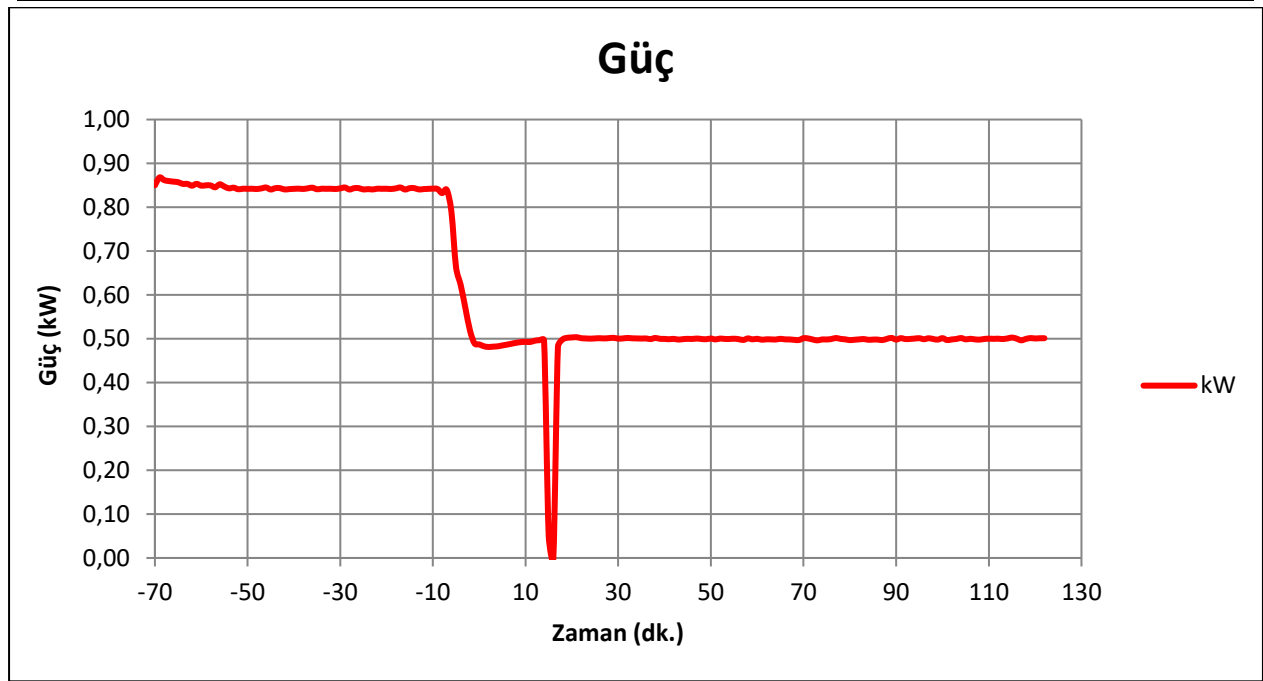
Şekil B5: Test esnasındaki motor gücü ölçümü
