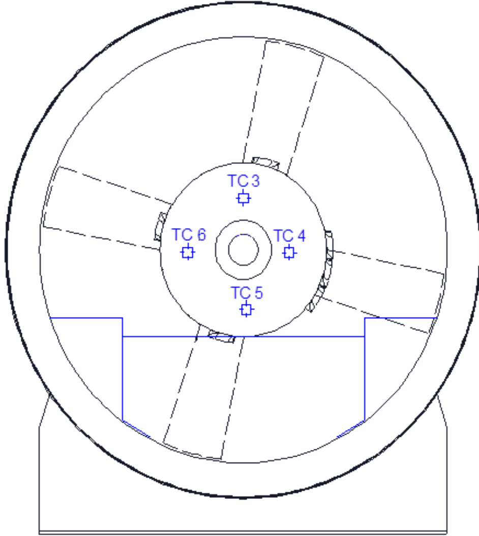
Şekil B1: Motor karkası üstündeki ısı çiftlerinin konumu
