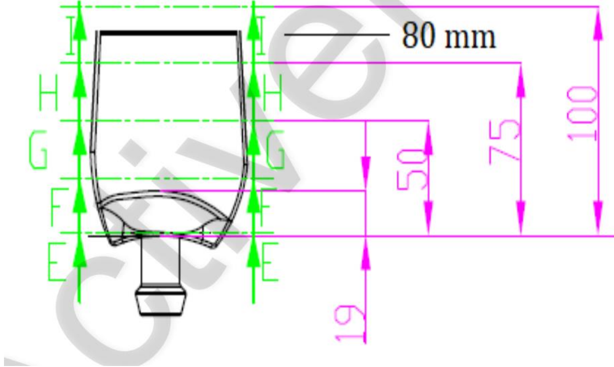
Şekil 4: Pervane boyut detayları.
