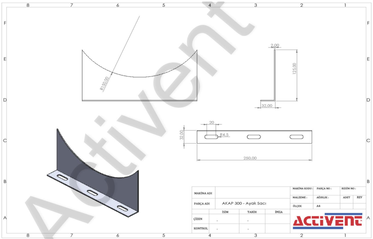
Şekil 7: Karkas destek ayağı detayları.
