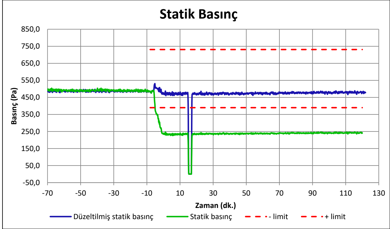
Şekil A2: Fanın ürettiği statik basıncı
